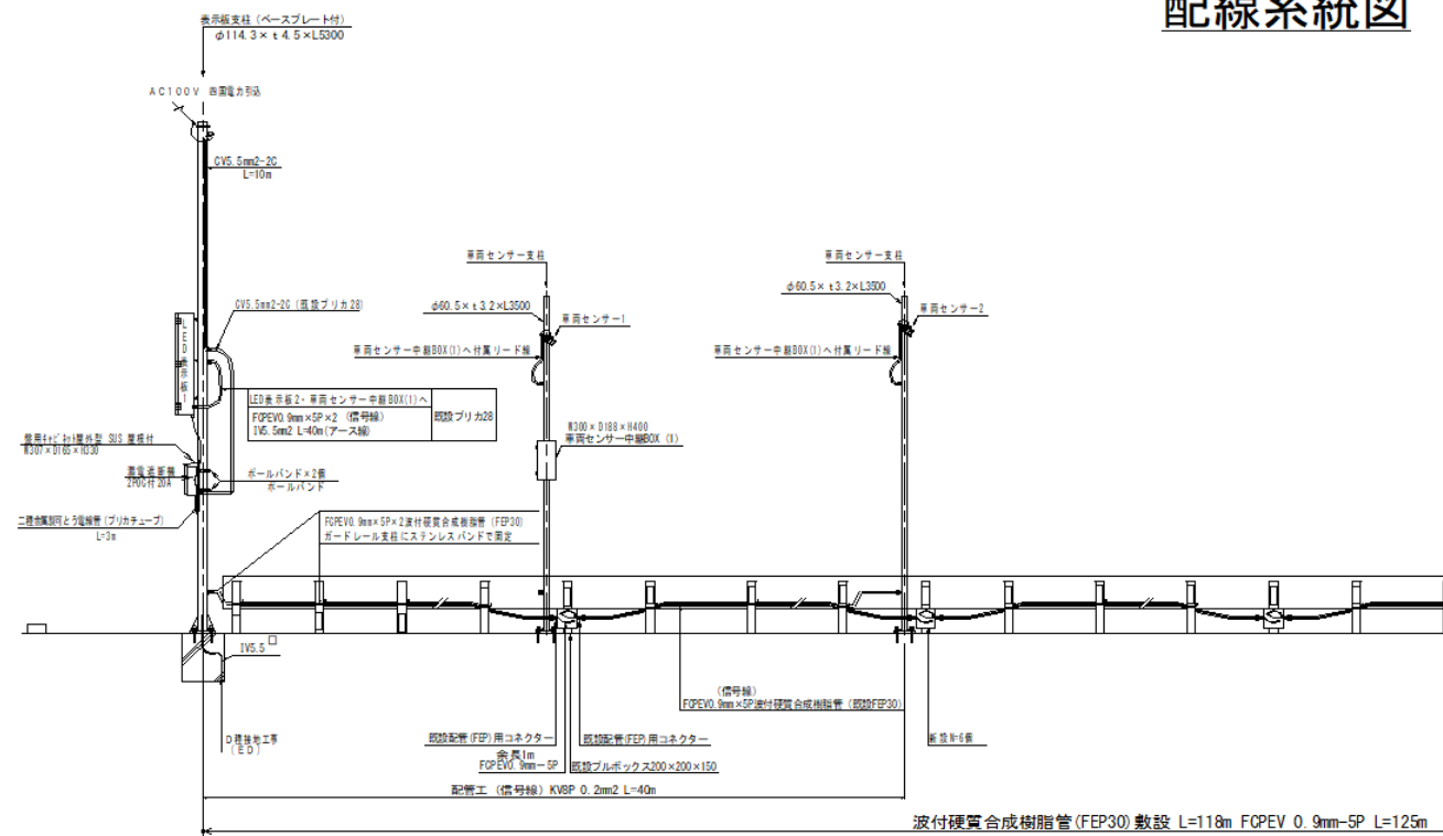
配線系統図
